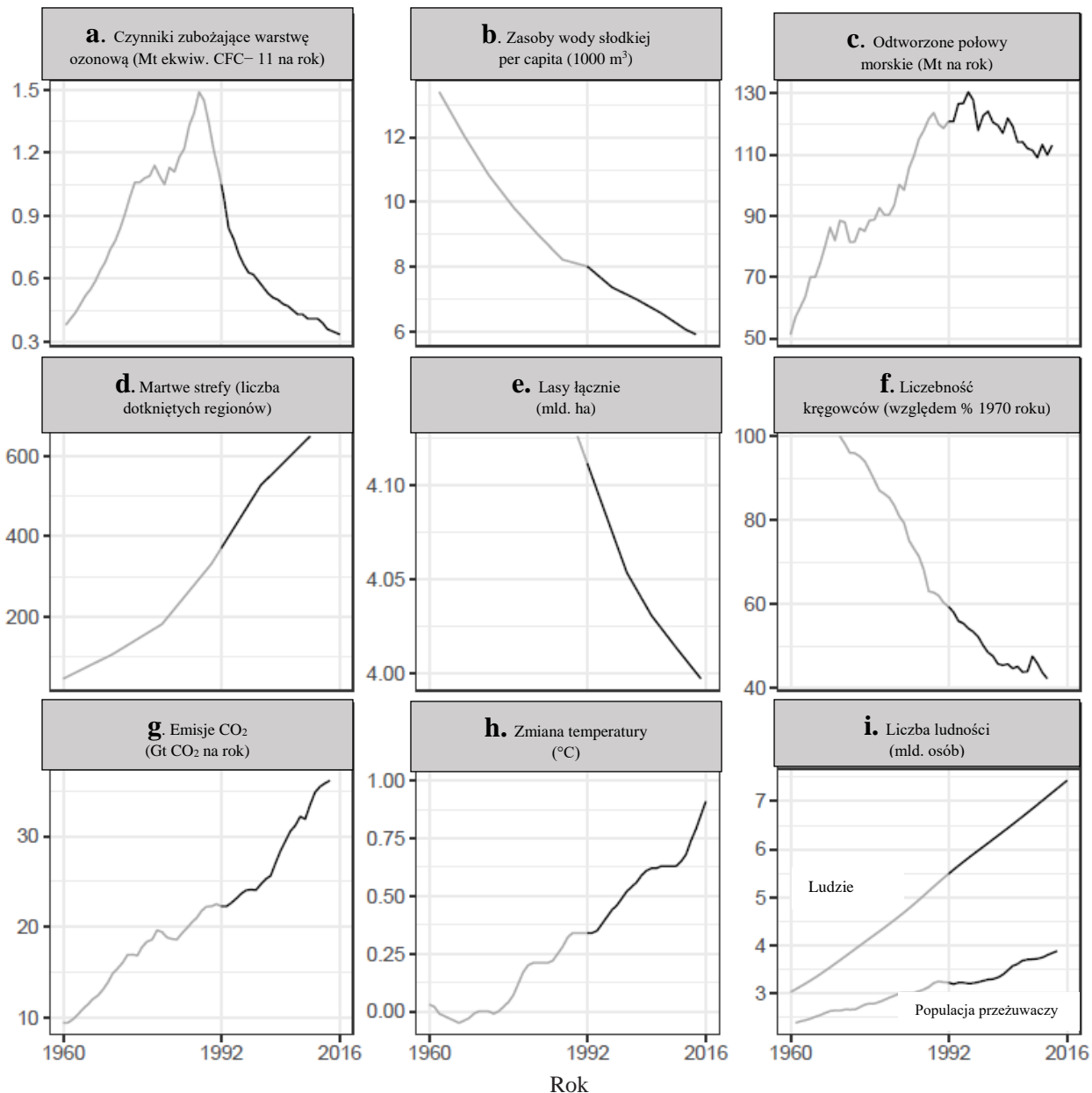
Rycina 1. Problemy środowiskowe zidentyfikowane w ostrzeżeniach naukowców dla ludzkości z 1992 roku w ujęciu czasowym. Lata przed i po ostrzeżeniu naukowców z 1992 roku oznaczono odpowiednio szarą i czarną linią. Rycina (a) pokazuje emisje gazów halogenowych, które niszczą ozon w stratosferze, przy założeniu stałego naturalnego współczynnika emisji 0,11 ton ekwiwalentu CFC -11 rocznie. Na ryc. (c) połowy morskie spadają od połowy lat 90. XX wieku, czemu towarzyszy wzrost wysiłku połowowego (plik uzupełniający S1). Wskaźnik liczebności kręgowców na ryc. (f) został skorygowany w celu wyeliminowania taksonomicznych i geograficznych błędów, obejmuje on stosunkowo niewiele danych z krajów rozwijających się, w których przeprowadza się najmniej badań; w latach 1970-2012 wystąpił 58-procentowy spadek liczebności kręgowców, w tym odpowiednio o 81, 36 i 35 procent dla populacji słodkowodnych, morskich i lądowych (plik S1). Średnie pięcioletnie pokazano w ryc. (h). Na ryc. (i) populacja przeżuwaczy obejmuje bydło domowe, owce, kozy i bawoły. Uwaga: osie Y nie rozpoczynają się od zera i konieczne jest sprawdzenie zakresu danych przy interpretacji każdego wykresu. Zmiana procentowa od 1992 roku dla zmiennych w każdym panelu kształtuje się następująco: (a) -68,1%; (b) -26,1%; (c) -6,4%; (d) +75,3%; (e) -2,8%; (f) -28,9%; (g) +62,1%; (h) +167,6%; oraz (i) ludzie: +35,5%, populacja przeżuwaczy: +20,5%. Dodatkowe opisy zmiennych i trendów, a także źródła dla ryciny 1, są zawarte w pliku S1.
